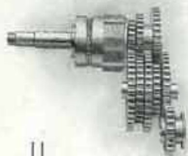
Cambio di Velocità e frizione (brevettato)
