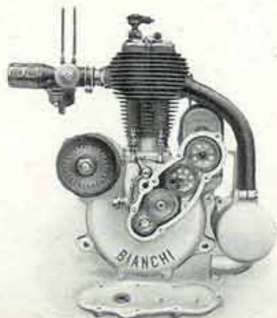
Interno e disposizione dei Comandi valvole e Magnete
